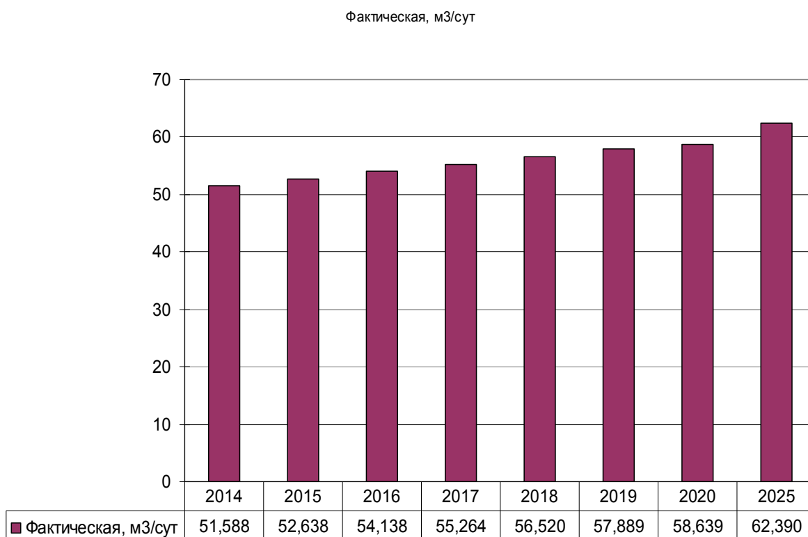
Рисунок 22 – Прогноз перспективного среднесуточного потребления воды д. Пушкири
