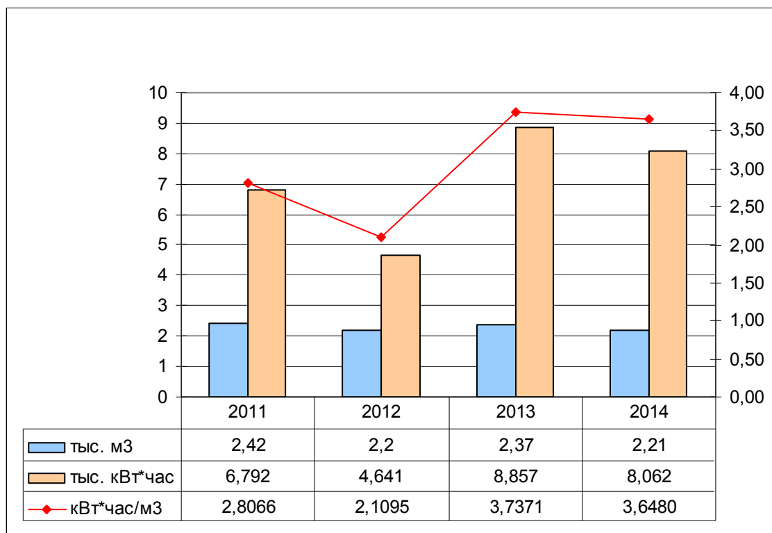
Рисунок 6 – Динамика изменения объемов потребления энергоресурсов скважиной №1586 д.М.Ошворцы 59а за период с 2011-2014 гг.
