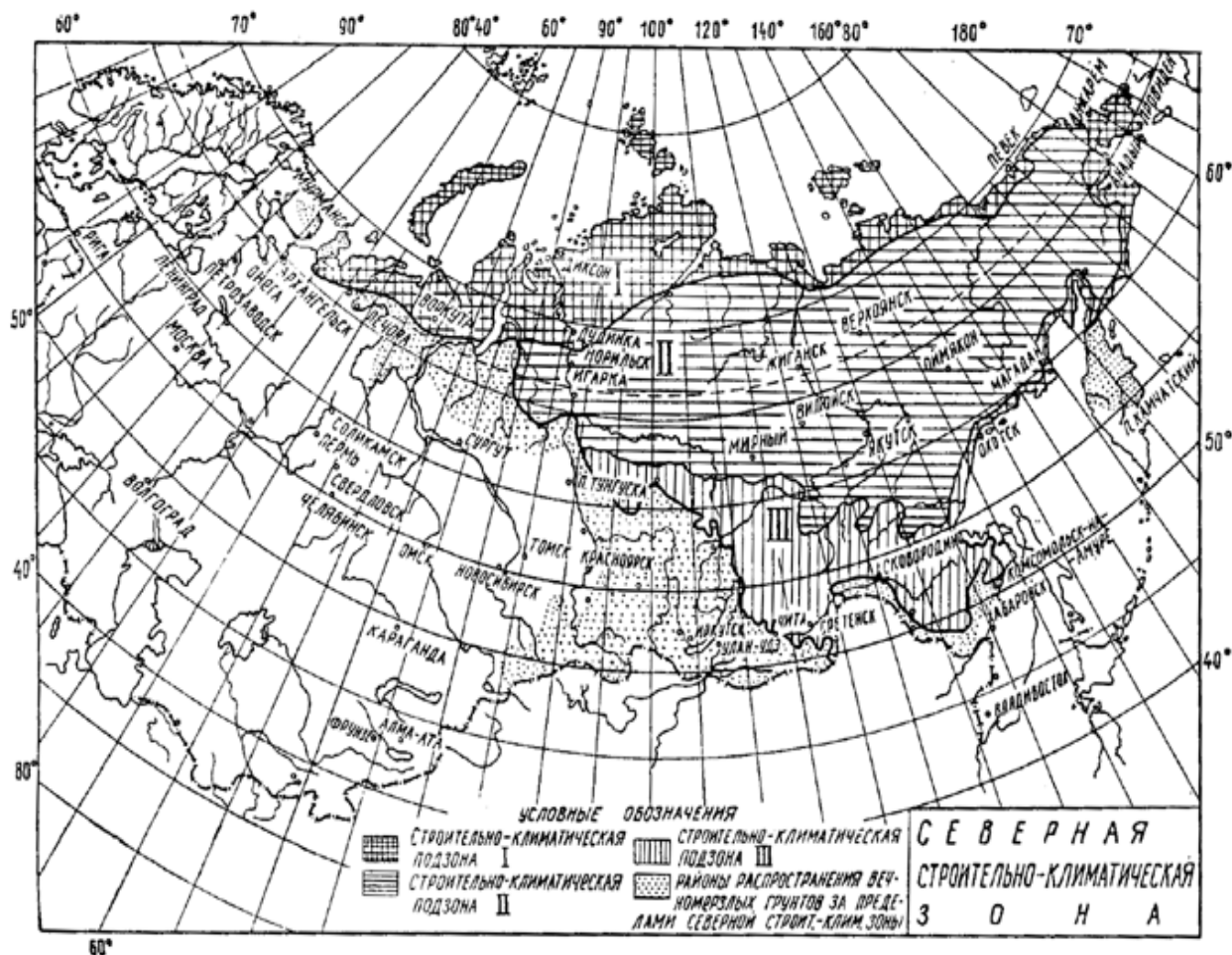
Рисунок 9 – Схематическая карта распространения вечномёрзлых грунтов и сейсмичности
