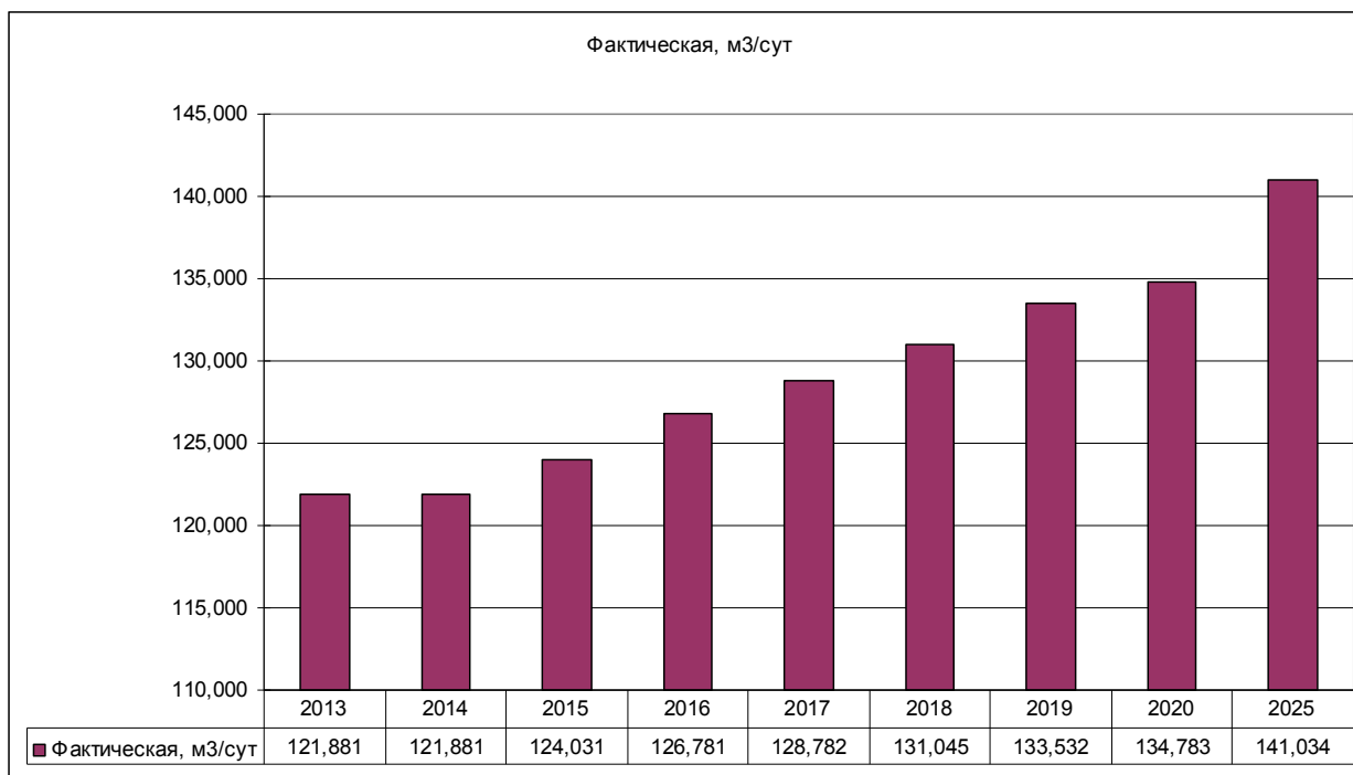
Рисунок 25 – Прогноз перспективного среднесуточного потребления воды МО «Пушкаревское»
