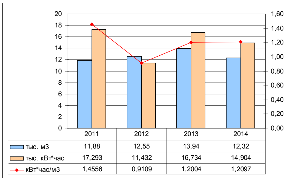
Рисунок 4 – Динамика изменения объемов потребления энергоресурсов скважиной №1003 д.Пушкари ул.Новая за период с 2011-2014 гг.
