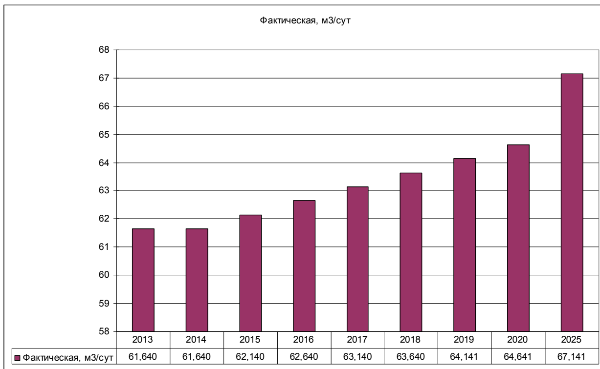
Рисунок 23 – Прогноз перспективного среднесуточного потребления воды с. Маяк
