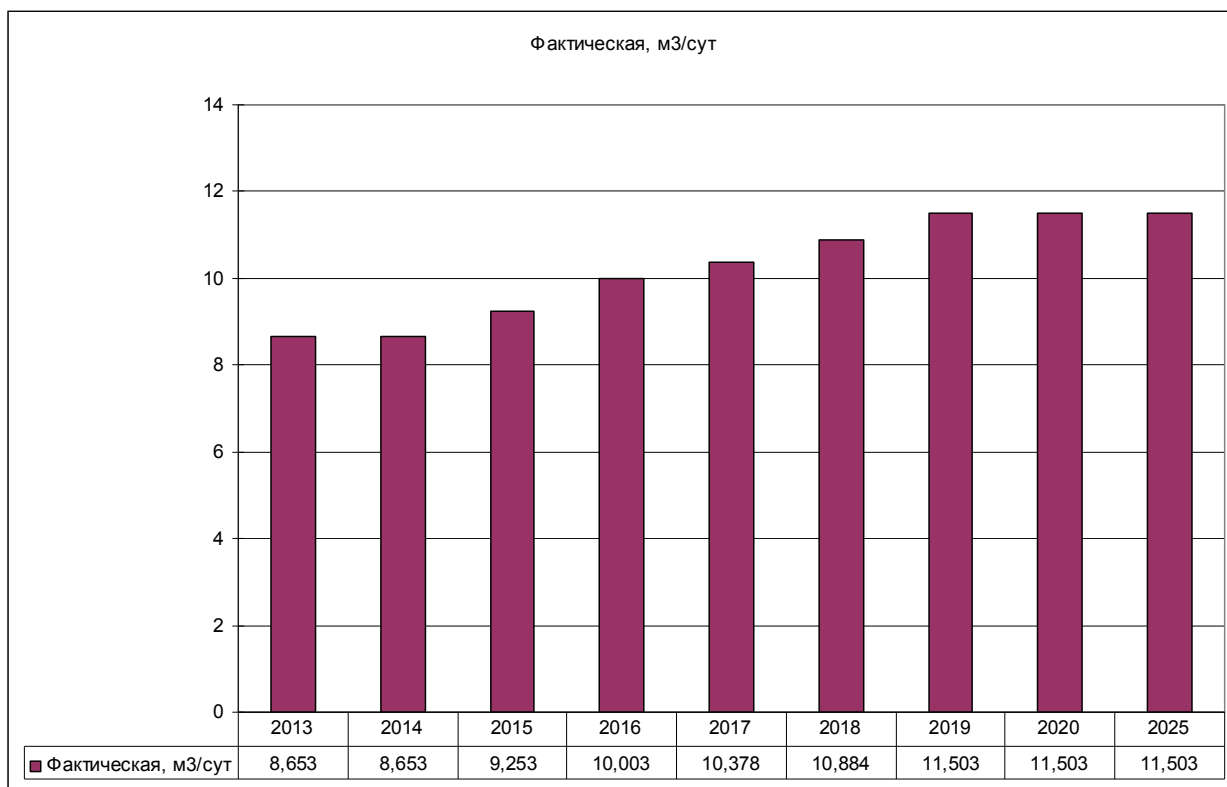
Рисунок 24 – Прогноз перспективного среднесуточного потребления воды д. М. Ошворцы
