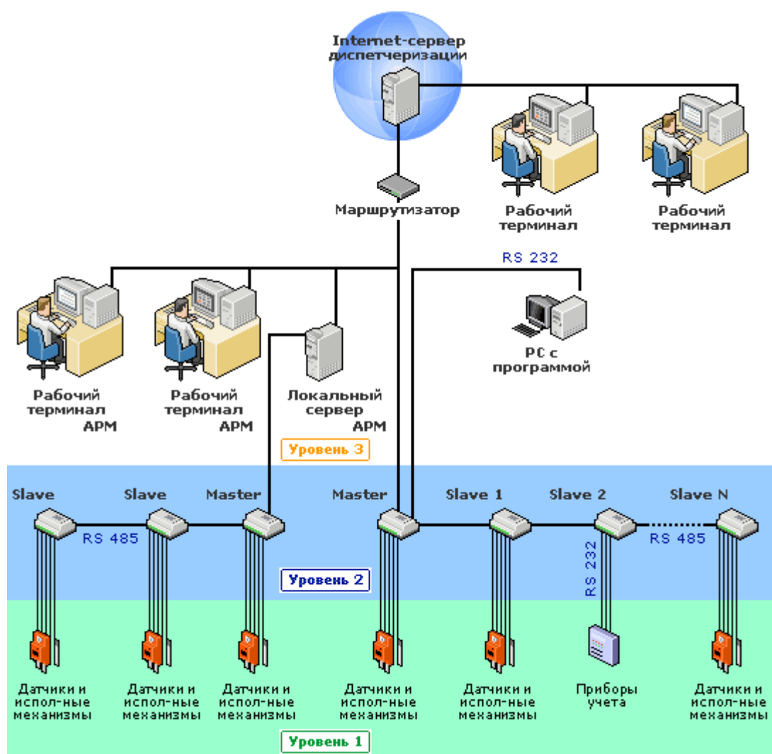
Рисунок 27 – Схема уровней системы АСУ ТП
