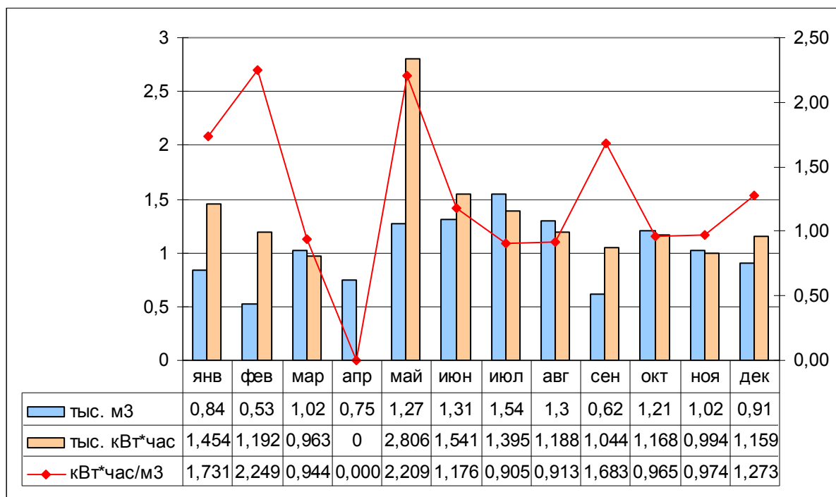
Рисунок 5 – Динамика сезонного изменения объемов потребления электроэнергии скважиной №1003 д.Пушкари ул.Новая за 2014 г.
