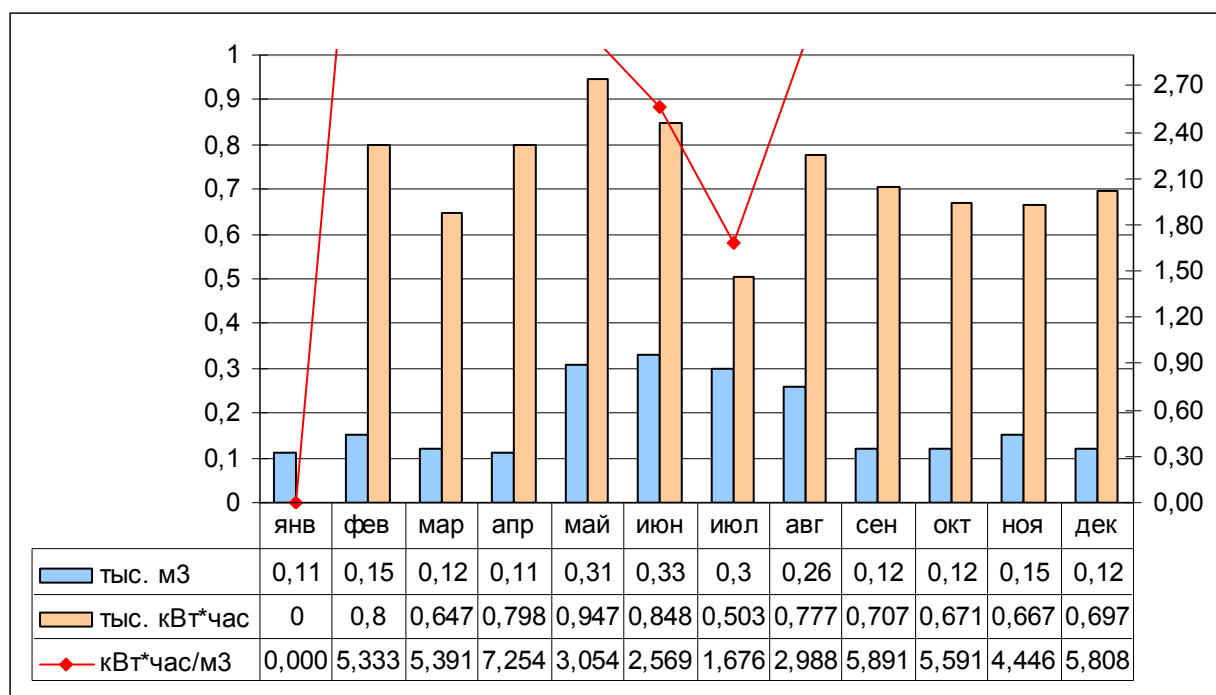
Рисунок 7 – Динамика сезонного изменения объемов потребления электроэнергии скважиной №1586 д.М.Ошворцы 59а за 2014 г.
