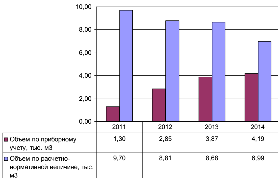
Рисунок 19 – Динамика изменения объемов потребления воды по фактическим и расчетным данным за период с 2011 по 2014 гг.
